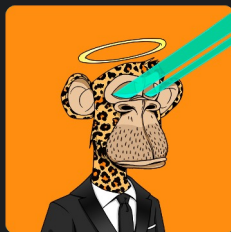
NFT
